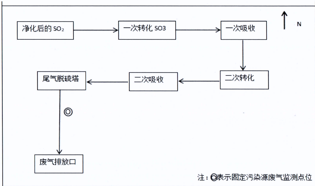
图3-1 废气监测点位示意图
